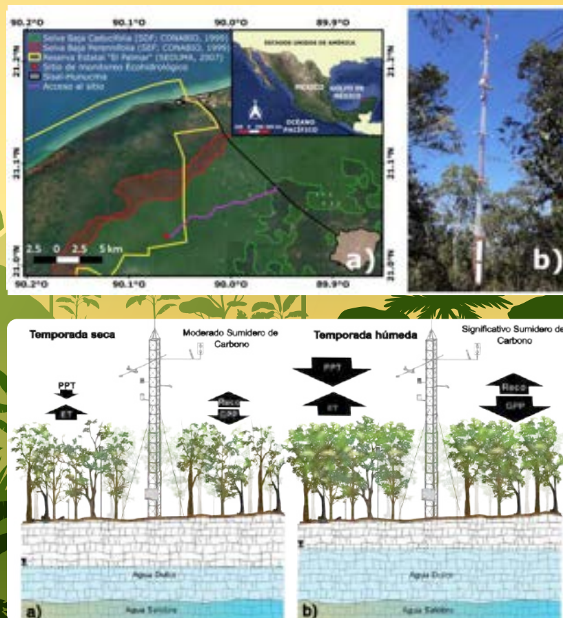
Figura 3. Diagrama conceptual de los flujos diurnos para la época seca y húmeda del año. PPT: Precipitación; ET: Flujo de vapor de agua (Evapotranspiración); GPP: Captura de \text{CO}_2 vía fotosíntesis (Producción Primaria Bruta); Reco: Liberación a la atmósfera de \text{CO}_2 vía la Respiración del Ecosistema.
